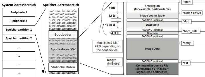
Abbildung 2.8: Memory Mapping mit Betrachtung eines Codeblockes nach [4] und [5]
