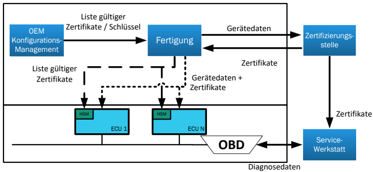
Abbildung 3.4: Konzeptionierung zur Authentifizierung und Autorisierung von Steuergeräten und Software zueinander nach Mundhenk [9]
