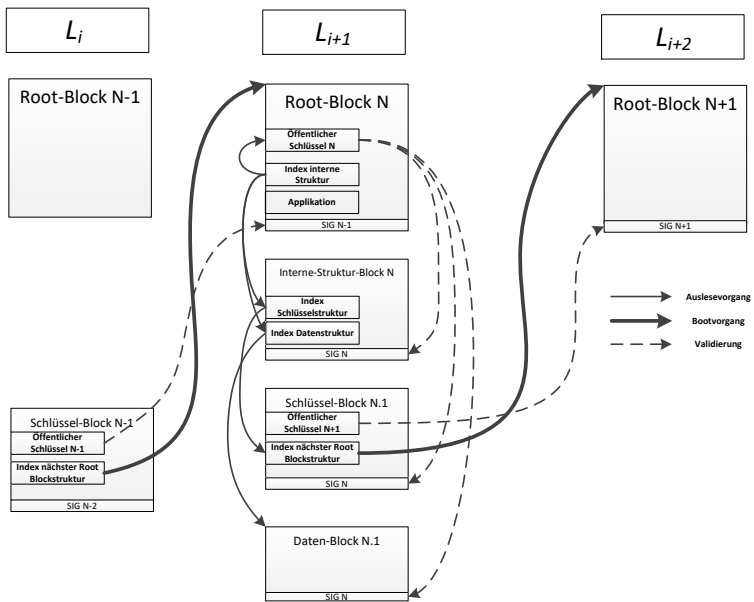
Abbildung 5.9: Bootabfolge einer Instanz
