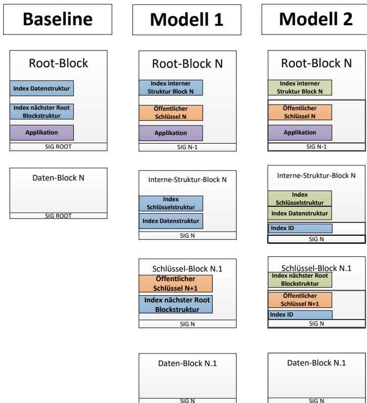
Abbildung 6.2: Sicherheitsrelevante Systemkomponenten
