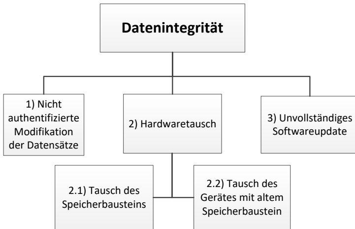
Abbildung 6.4: Angriffsbaum Datenintegrität
