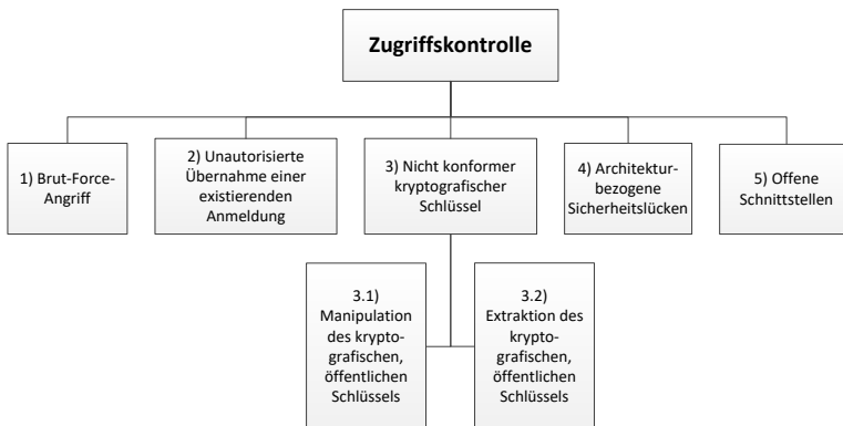
Abbildung 6.3: Angriffsbaum „Zugriffskontrolle“
